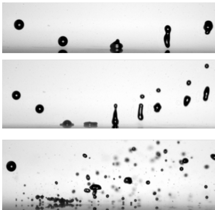
Impact de gouttes sur une paroi à haute température
