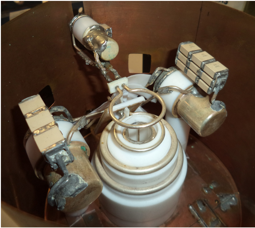
Bobine radiofréquence pour la spectroscopie RMN dans les matériaux à temps de relaxation courts
