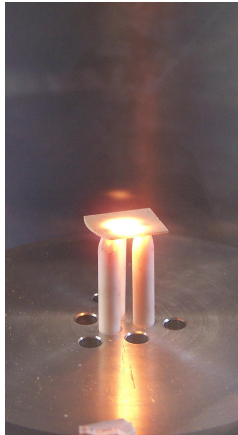
Étude d'un échantillon d'oxyde de titane à haute température
