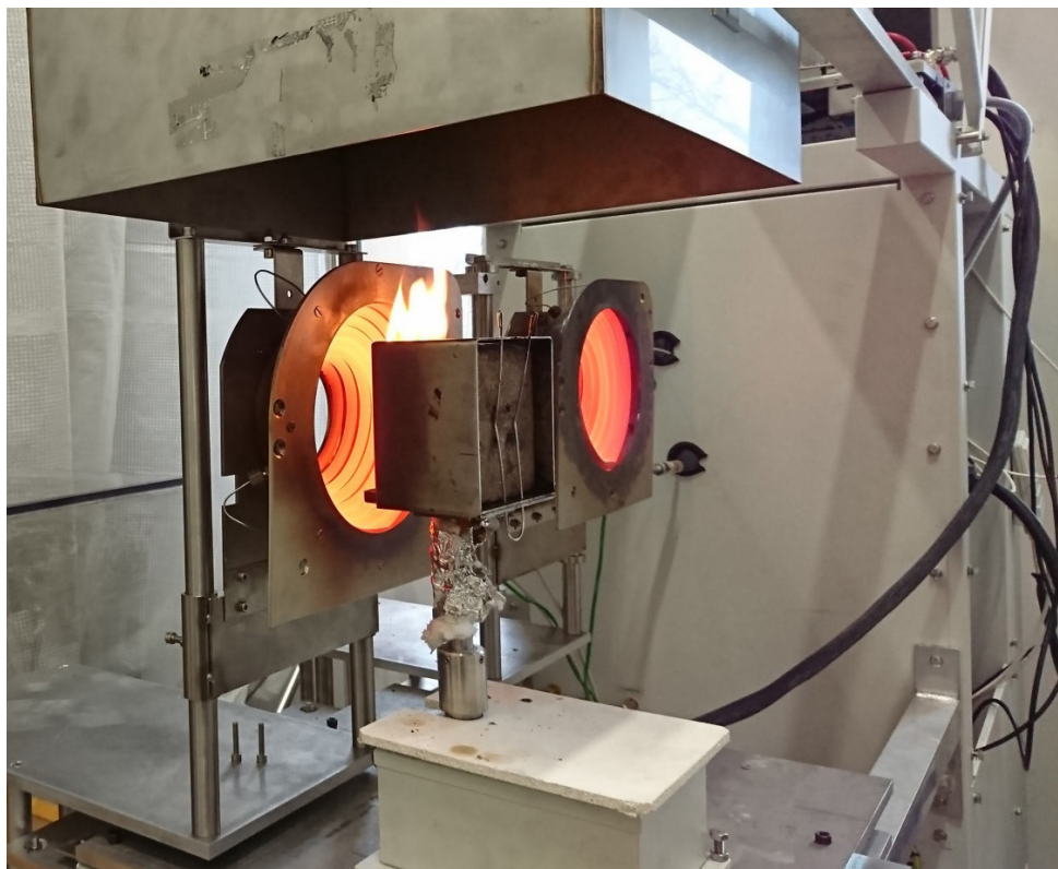
Essai sur l'inflammabilité du bois sous des conditions de flux thermiques donnés
